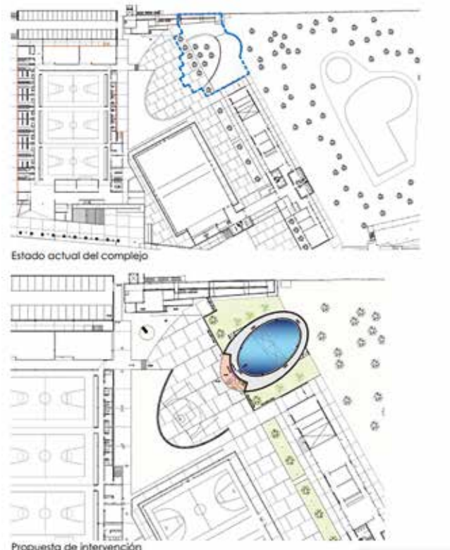
Fotografía: Plano de la ampliación de la piscina de verano.
